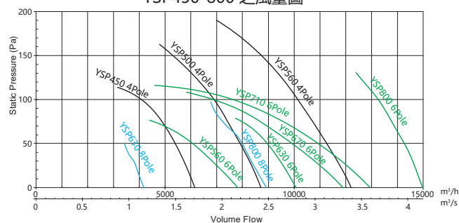
YSP450-800 之風量圖
